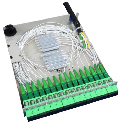
Simulação da montagem com cabo de entrada, pigtaills e adaptadores ópticos
