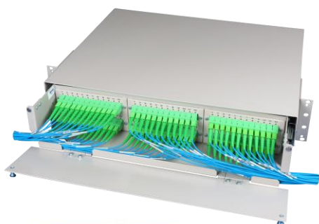
Saída frontal dos cordões de manobra (modelo 72 fibras)
