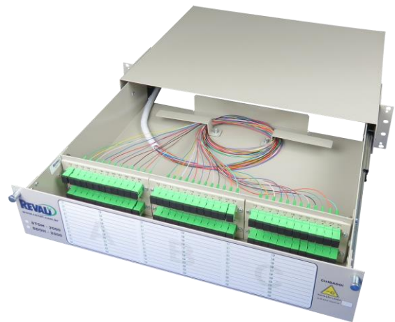
Acomodação interna das fibras e dos adaptadores ópticos (modelo 72 fibras)
